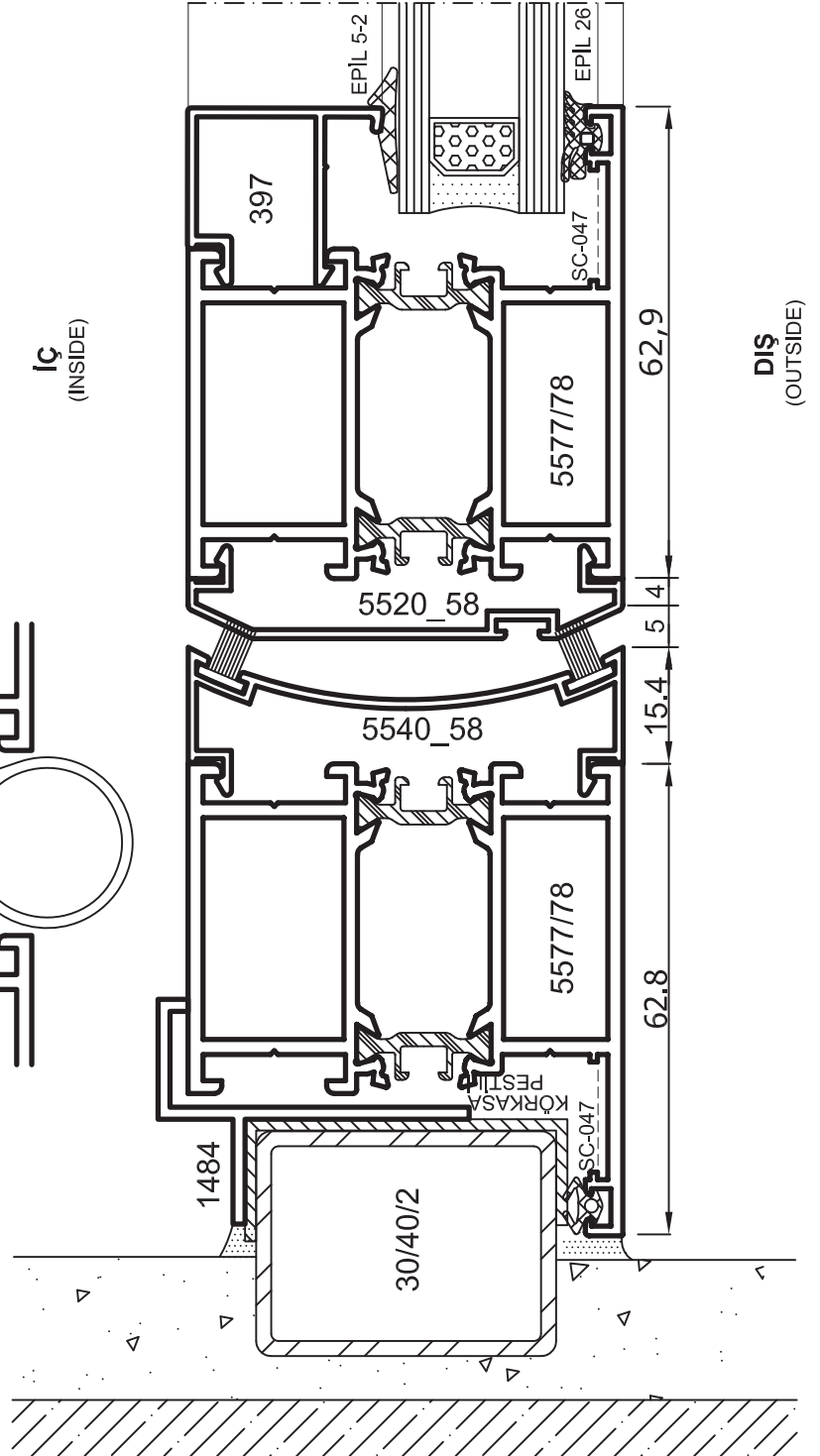
ÇARPMA KAPI SWING DOOR
