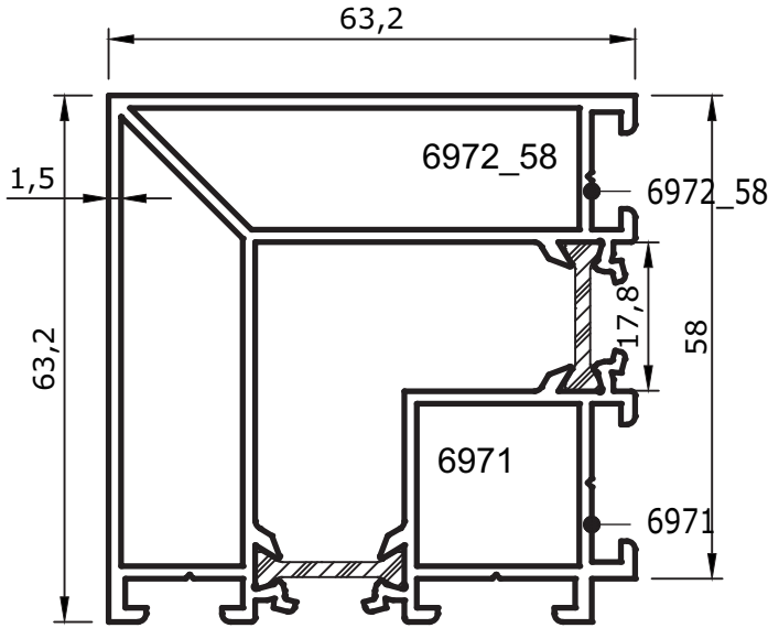
No:6971/72_58 90° Köşe Dönüş Profili 1,950 kg/m
