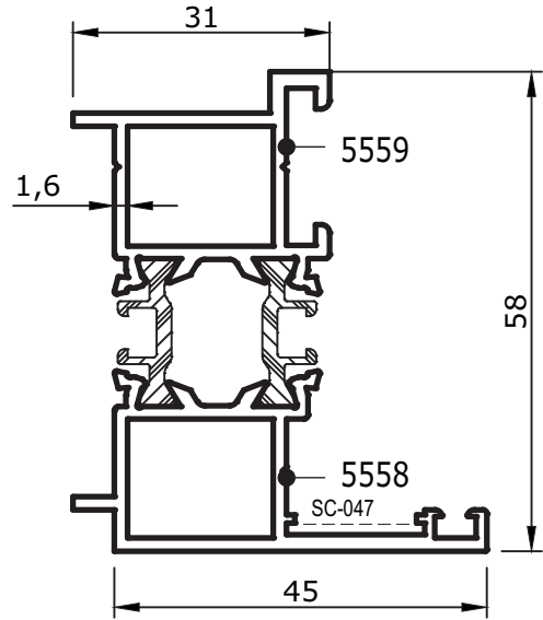
No:5558/59 Dışa Açılır Kapı Adaptörü 1.225 kg/m
