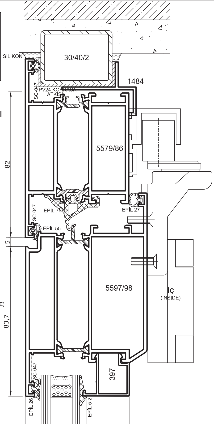
Folding Sliding System Detail Katlanır Kapı Sistem Detayı
