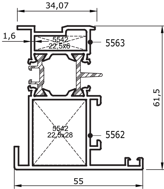
No:5562/63 Pivot Adaptörü 1,390 kg/m
